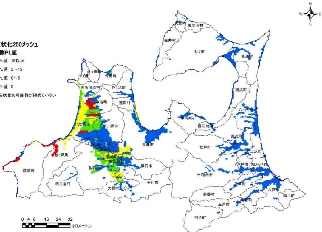
<図(2)-2 液状化危険度分布図>
