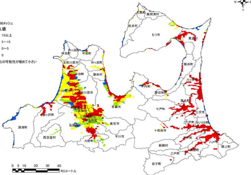
<図(1)-2 液状化危険度分布図>
