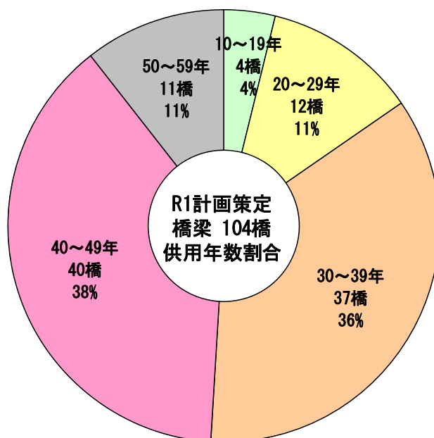
図 3-2 建設後経過年数別の割合
