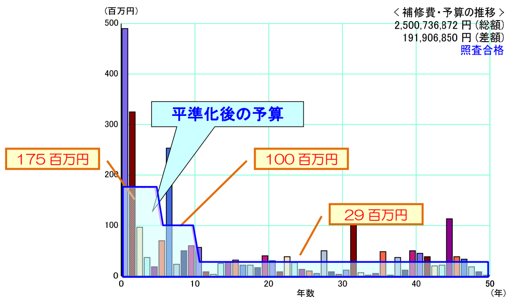
図 5-14 予算制約を考慮した予算シミュレーション結果
