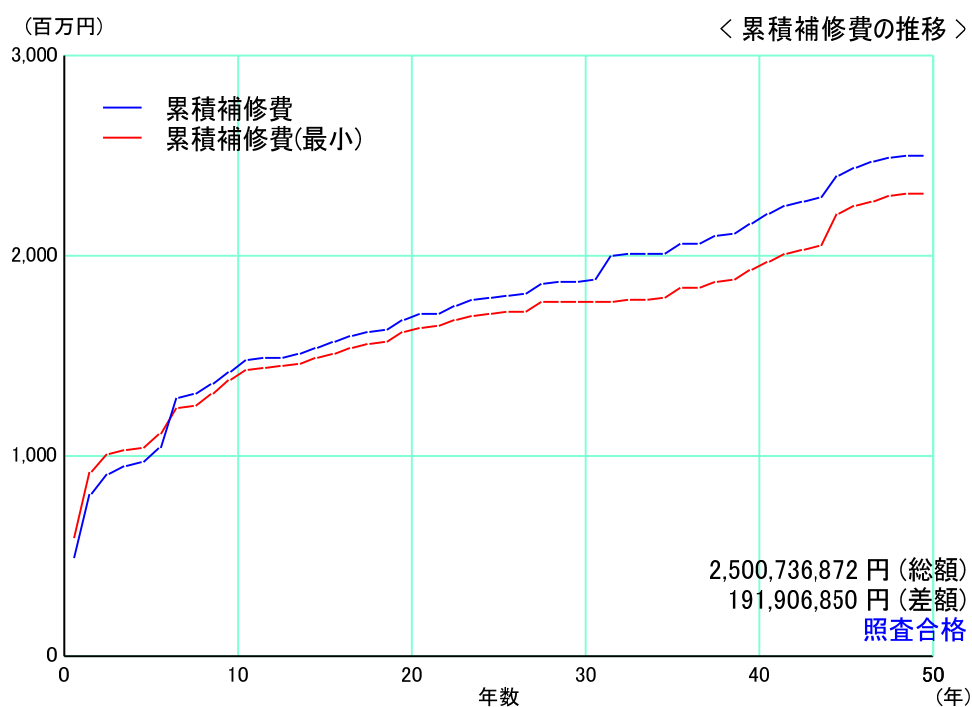
図 5-15 予算シミュレーション結果による累計補修費の推移
