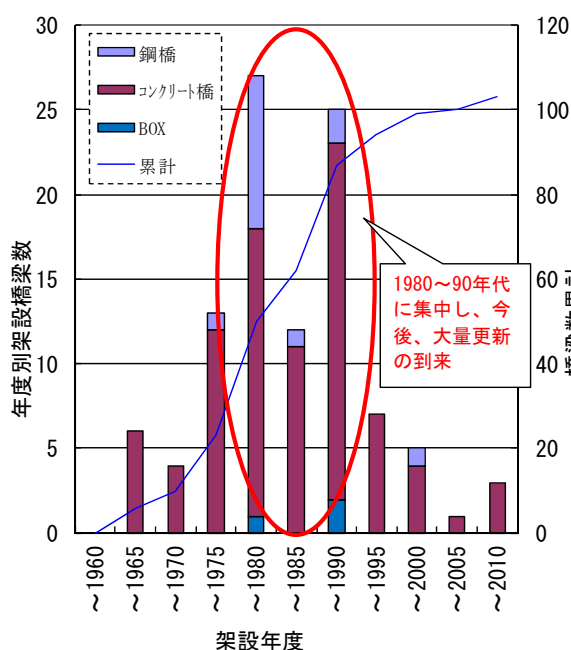
図 1-1 黒石市橋梁の状況
