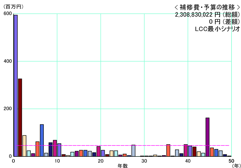
図 5-13 50 年間 LCC が最小となるシナリオの組合せにおける補修費の推移
