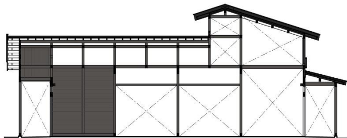
駐輪場側からの断面図
