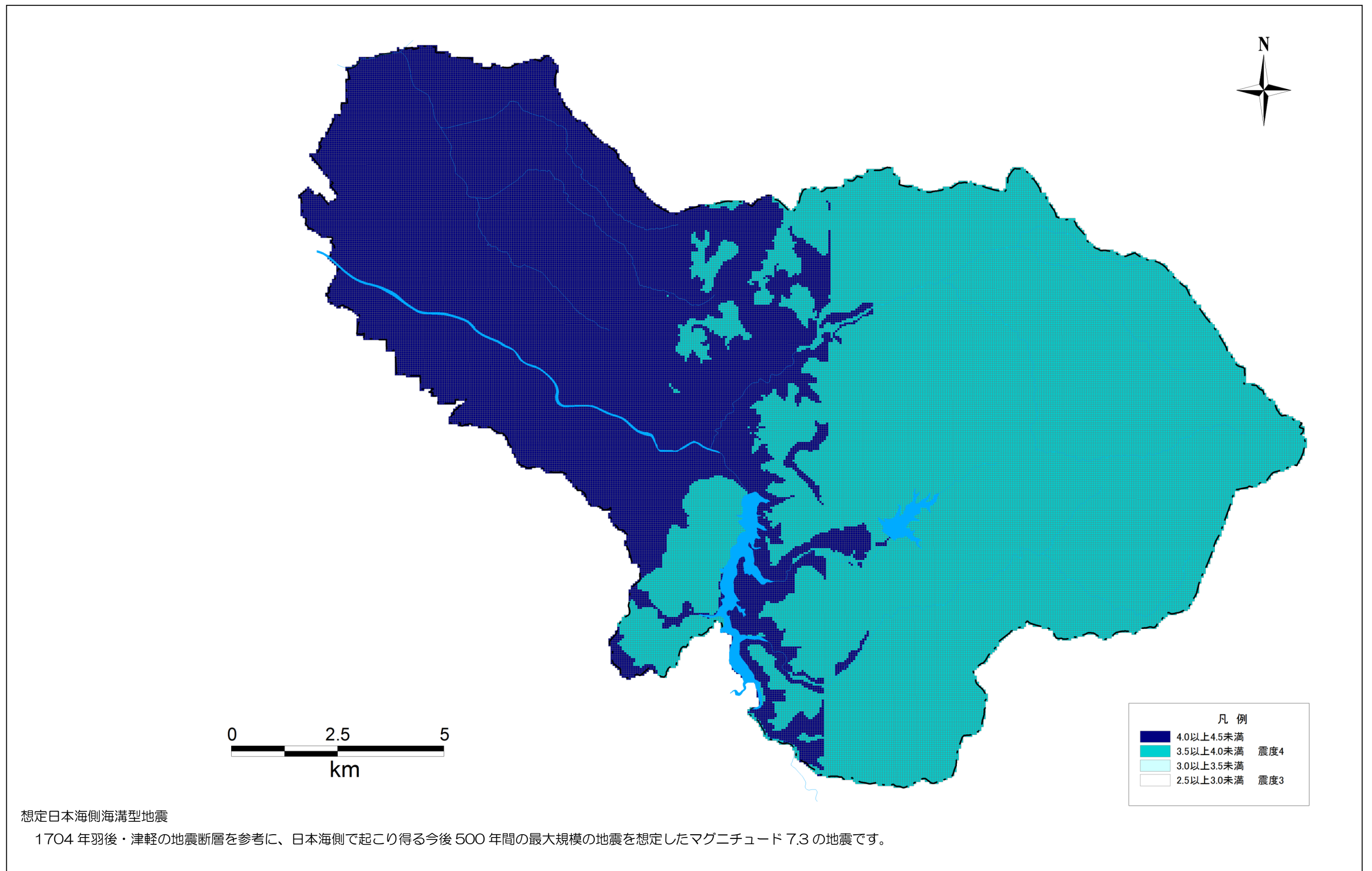
日本海側海溝型地震を想定した震度分布図
